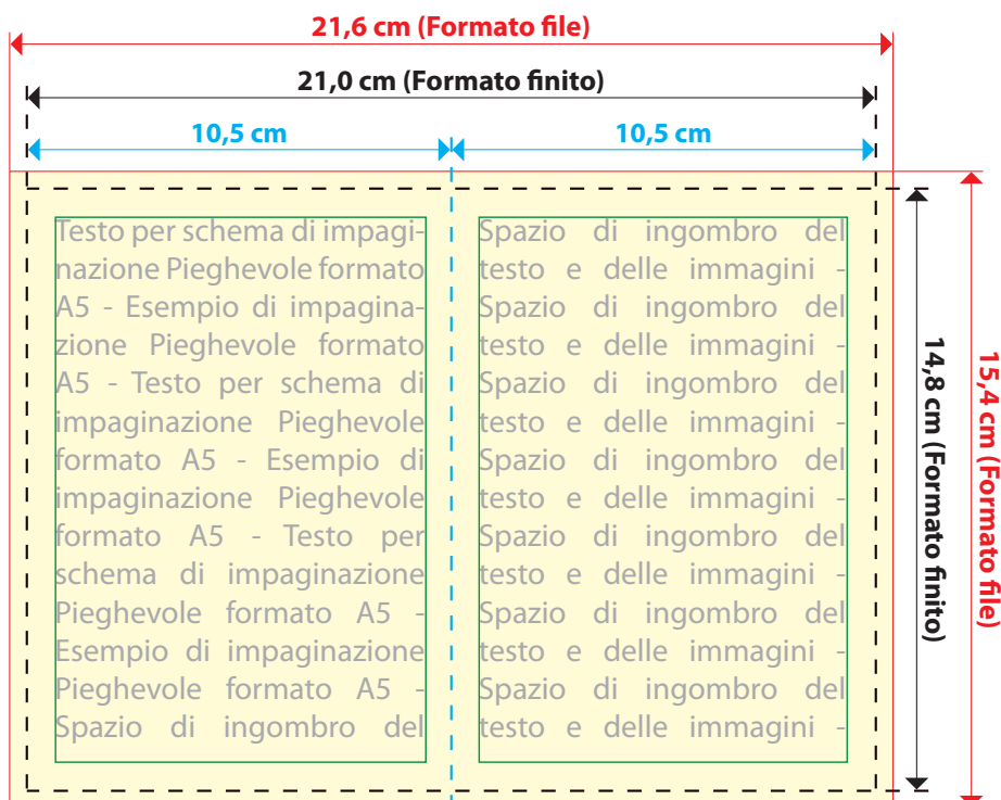
Vista dell' INTERNO dello stampato aperto
